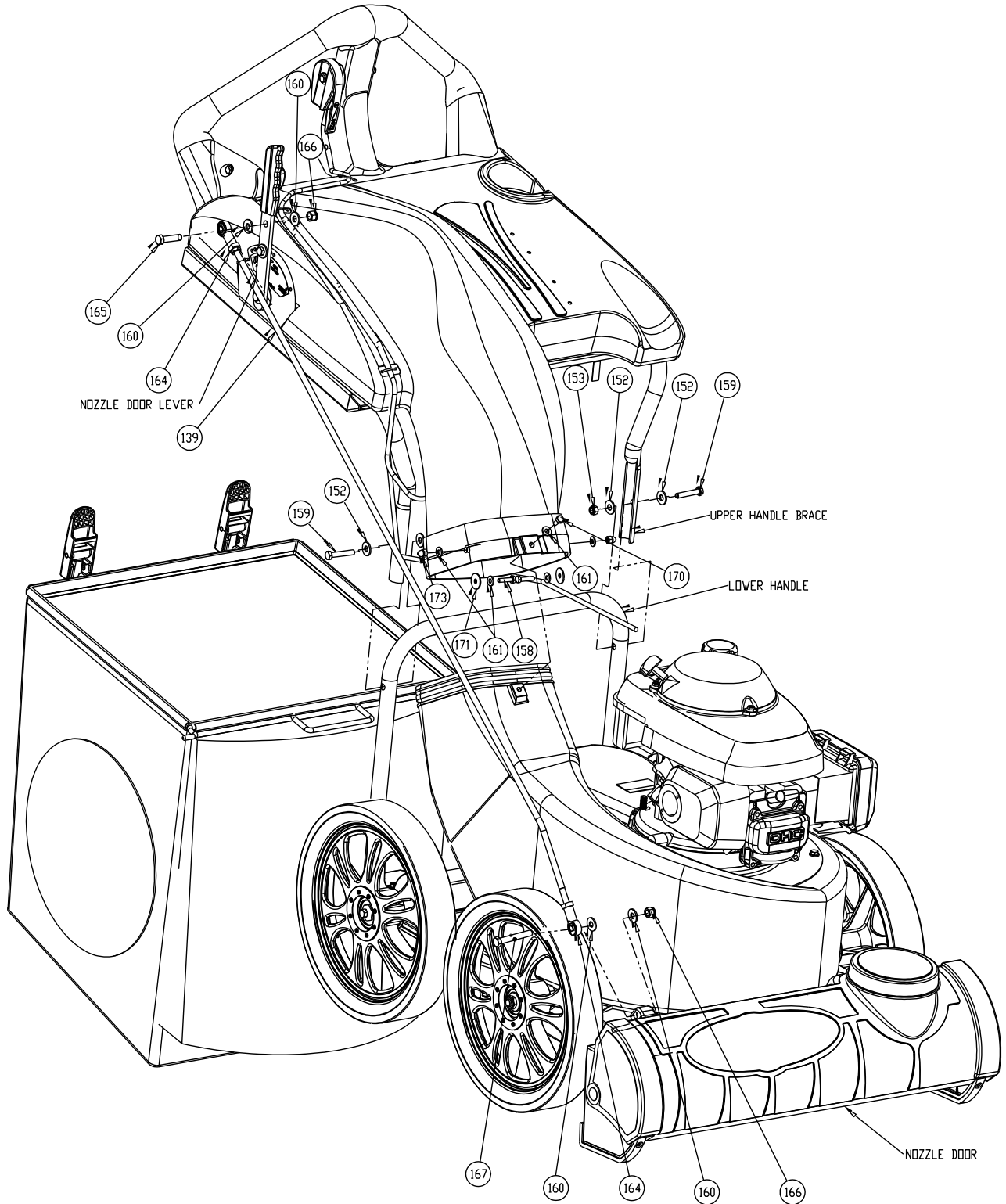
MV Sauger Bausatz Zeichnung
